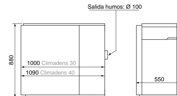
Conexiones y otras dimensiones consultar pág. 96 Accesorios y dimensionado chimenea consultar pág. 94
