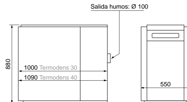
Conexiones y otras dimensiones consultar págs. 99 Accesorios y dimensionado chimenea consultar pág. 94
