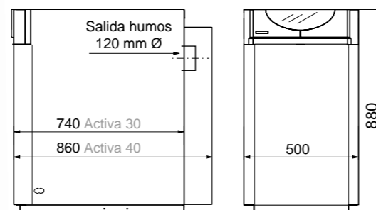
Conexiones y otras dimensiones consultar pág. 98
