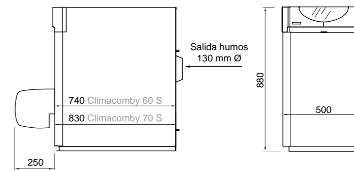
Conexiones y otras dimensiones consultar pág. 99
