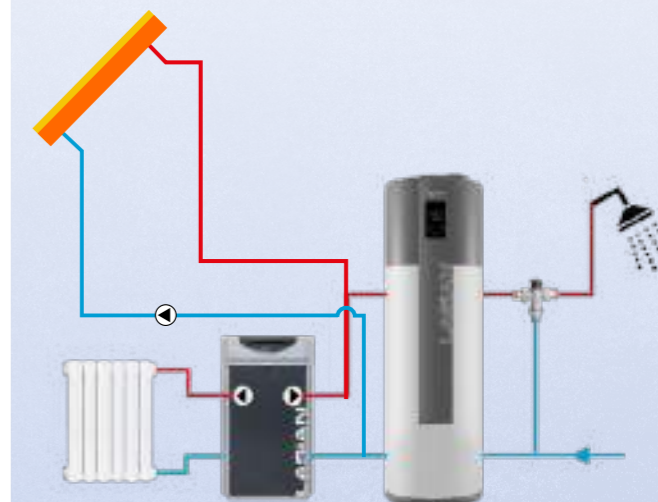
Esquema de funcionamiento de AQUARIA 250 S3 con una fuente de energía externa de apoyo de una caldera o energía solar.
