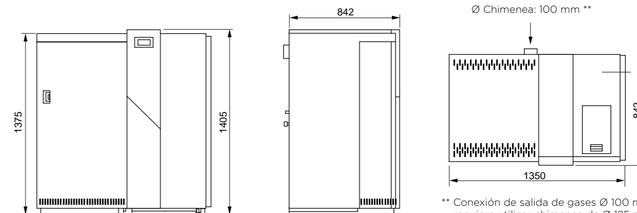
DIMENSIONES DE BIOMASTER 32 CON TOLVA DE 207 KG
