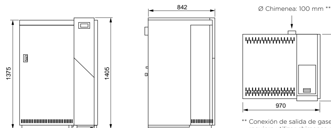
DIMENSIONES DE BIOMASTER 32 CON TOLVA DE 99 KG
